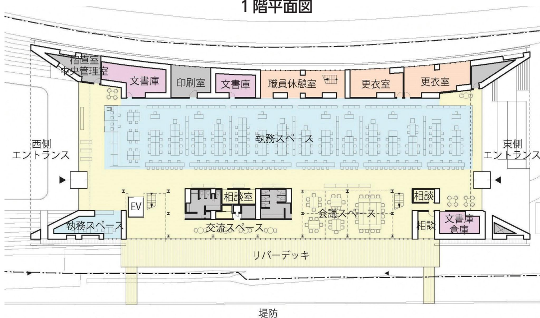
1階平面図
