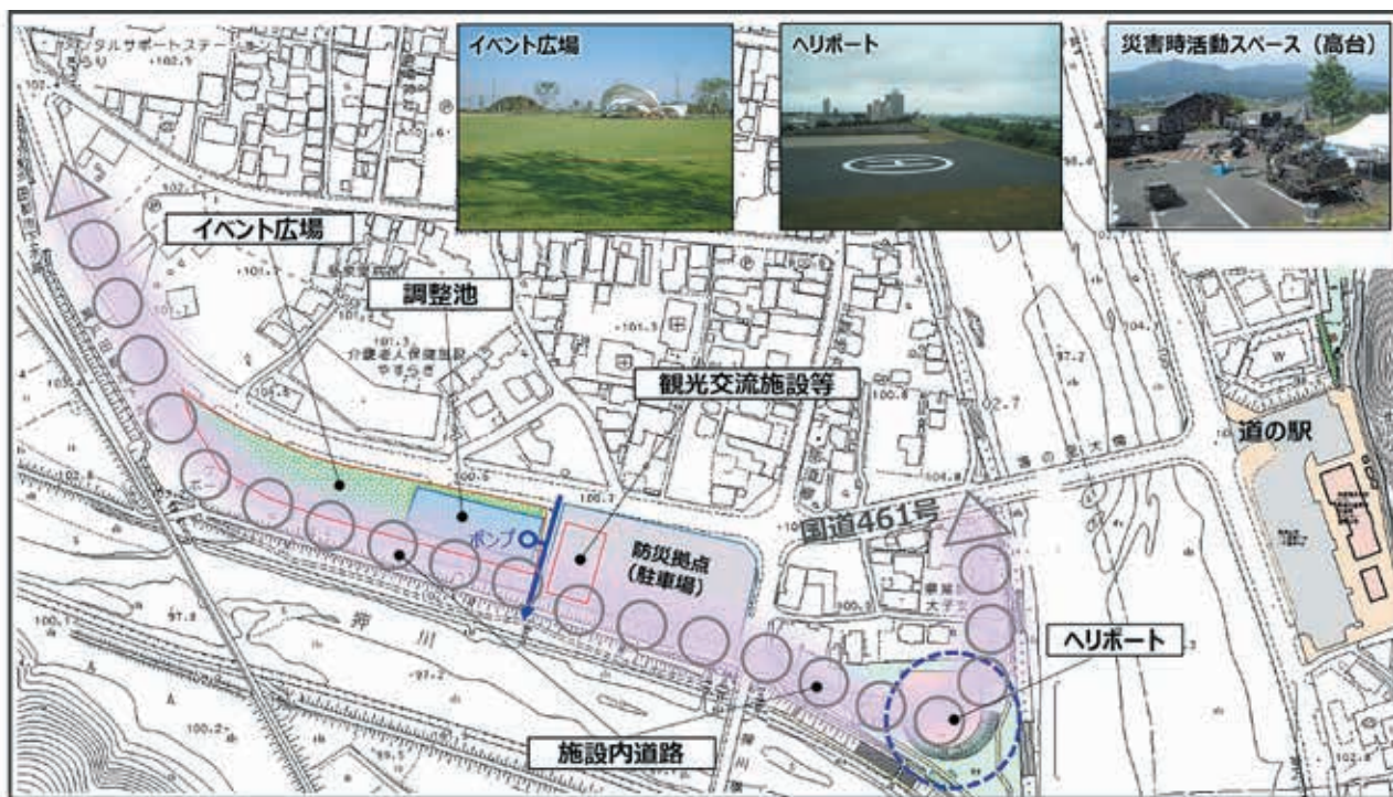
「防災道の駅」整備図面案
