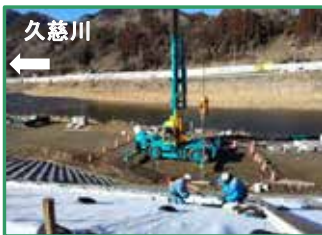
コンクリートブロックの設置を行っています
