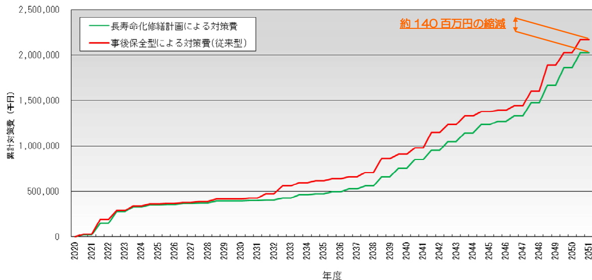
従来型維持管理と長寿命化修繕計画との累計対策費の比較
